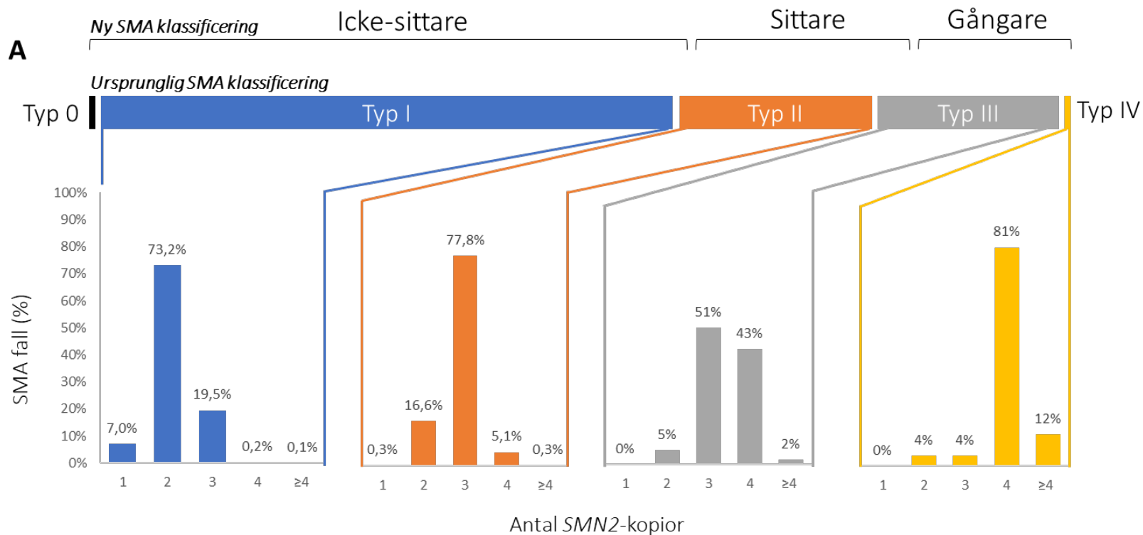
Figur 1 A och B. Figurerna visar på relationen mellan antal kopior på SMN2 -genen och de olika SMA typerna hos patienter som identifierats kliniskt. Siffrorna är baserade på en studie av Calucho och medarbetare (7) som sammanställt registerdata världen över. Figur A visar fördelningen av antal kopior på SMN2 -genen över de olika SMA typerna. Då det finns överlapp i motoriska färdigheter mellan de olika typerna av SMA har en alternativ indelning föreslagits: icke-sittare, sittare och gångare (anpassad från Wirth och medarbetare (3)) Figur B illustrerar fördelningen av SMA typer utifrån antalet kopior på SMN2 -genen.
