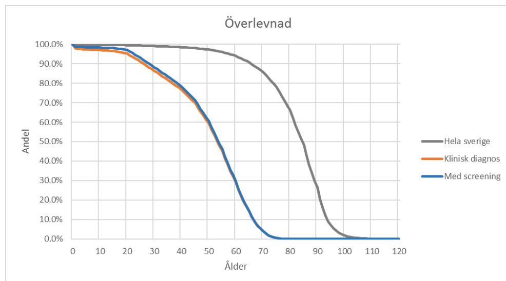
Figur 2: Beräknad överlevnad
