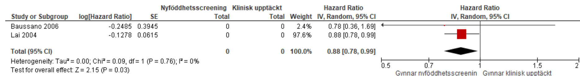
Träddiagram 5. Risk för infektion med P. aeruginosa
