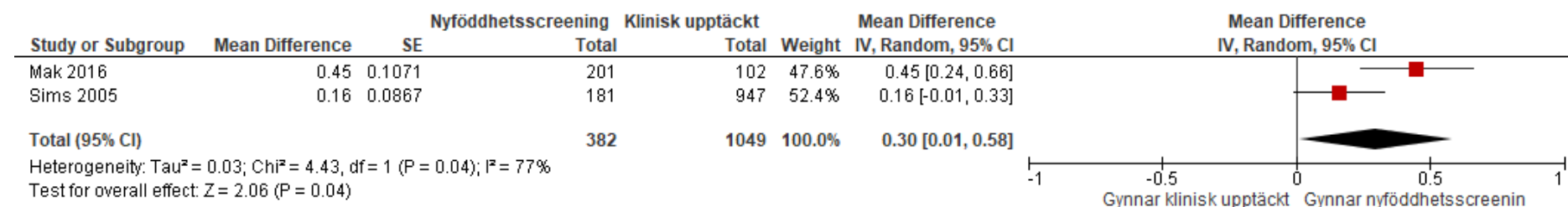
Träddiagram 3. Skillnad i z-värde över tid med avseende på vikt för åldern.
